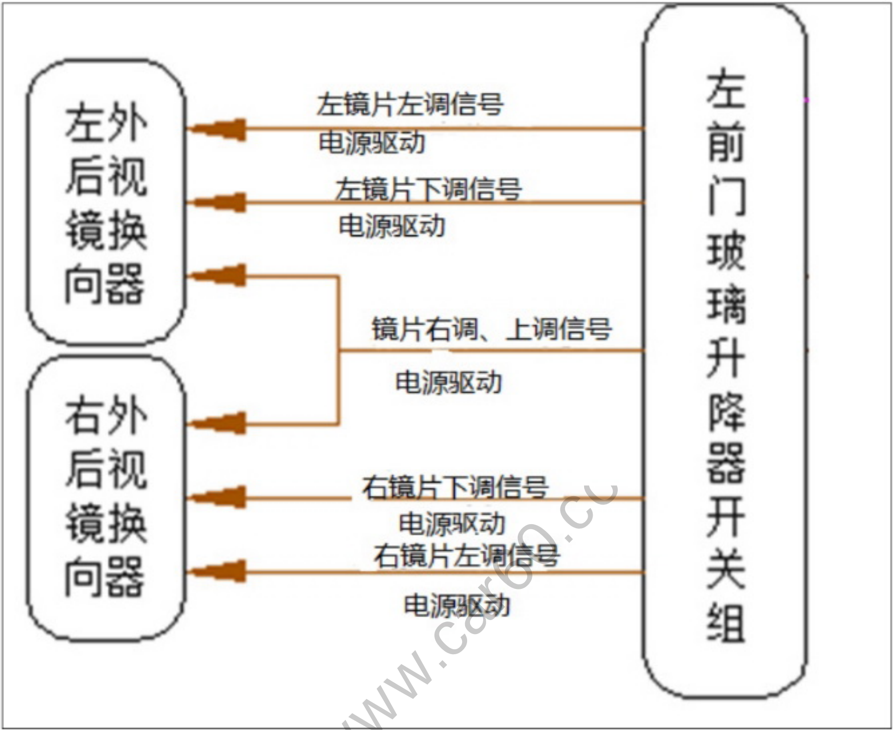
系统框图
